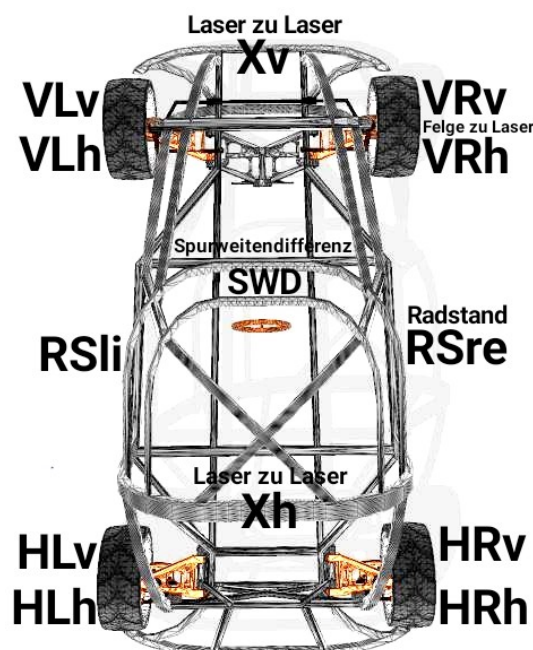
Abb. 2: Übersicht der Messwerte / Messorte (für Spurmessung)
