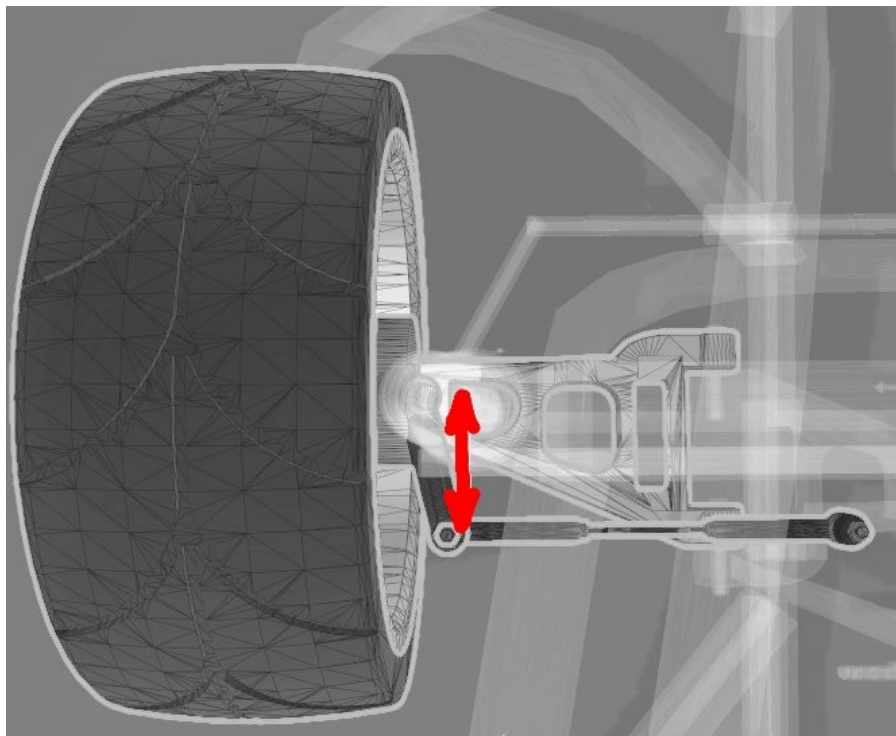
Abb. 1: Messen der Lenkhebel-Länge (Blick von oben)
