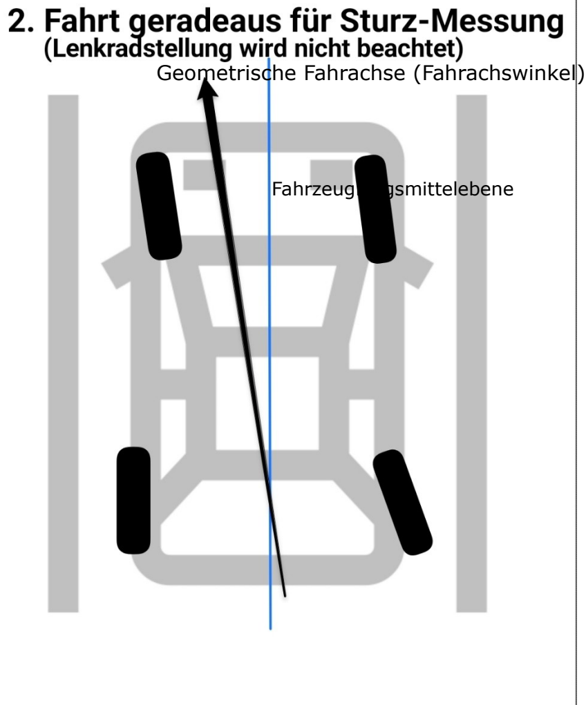
Abb. 5: Lenkradstellung -Fahrt geradeaus- (Hilfsstellung für die Sturzmessung)
