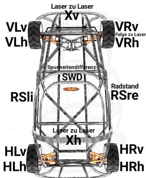
Abb. 2: Übersicht der Messwerte / Messorte (für Spurmessung)
